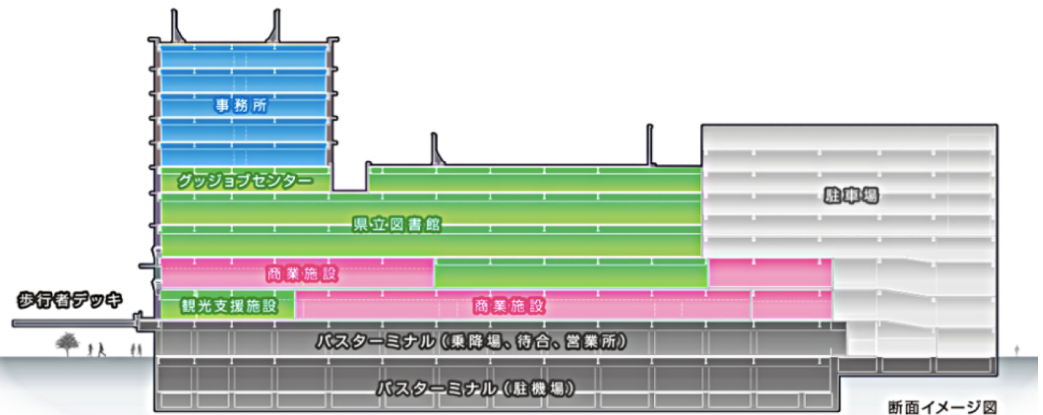
カフーナ旭橋A街区断面イメージ図 (カフーナ旭橋HPより)
